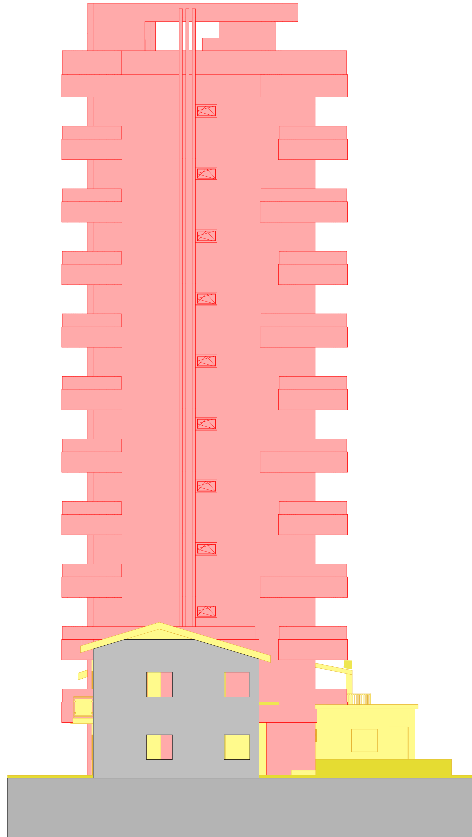
PROSPETTO OVEST - COMPARATIVA - SCALA 1:100
