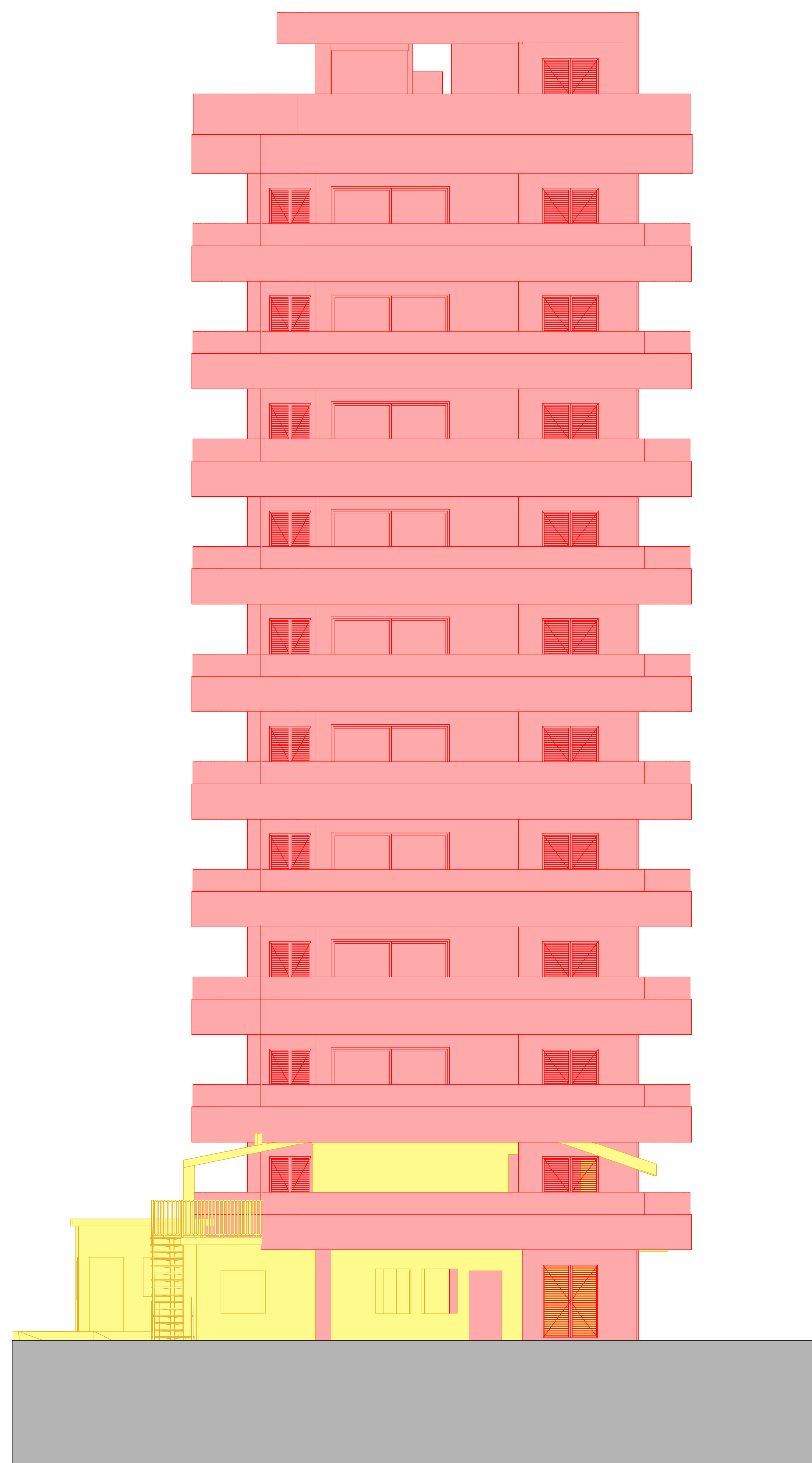
PROSPETTO EST - COMPARATIVA - SCALA 1:100
